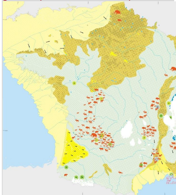
Figure 1. La France au dernier maximum glaciaire (18 000 ± 2 000 ans BP)
