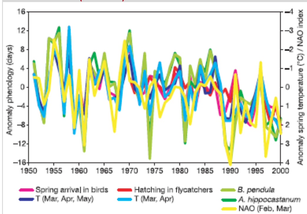
Figure 10. Évolution des anomalies temporelles des dates de quelques phénophases en relation avec deux variables climatiques, l'anomalie de température printanière et le North Atlantic Oscillation (Index Nao)
