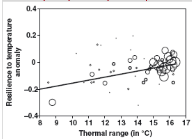
Figure 12. Relation entre la résilience à l'anomalie de température et l'amplitude thermique rencontrée par l'espèce sur la partie européenne de son aire de répartition
