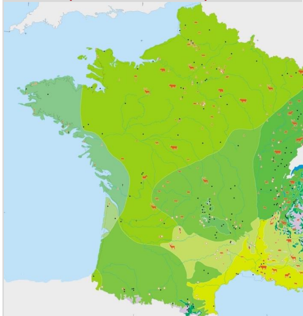
Figure 2. La France à l'optimum climatique holocène (8 000 ± 1 000 ans BP)
