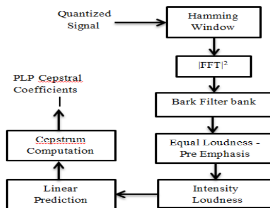
FIG. 5. PLP PARAMETER COMPUTATION
