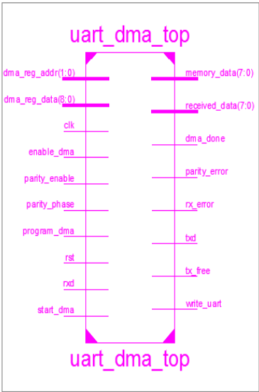
Fig 7: Top module
